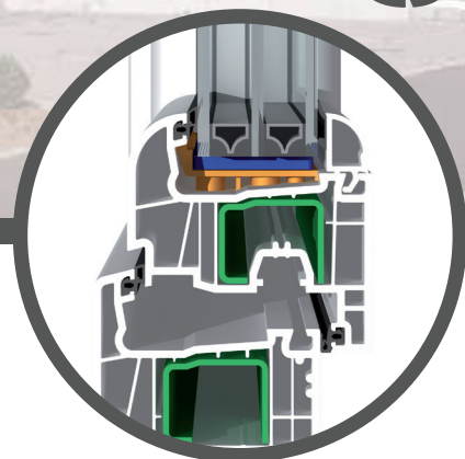
Streamline oblé krídlo
