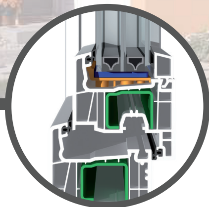
Streamline hranaté krídlo
